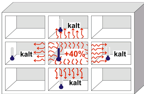
Abbildung 3: Transmissionswärme flüsse zwischen Wohnungen 11
